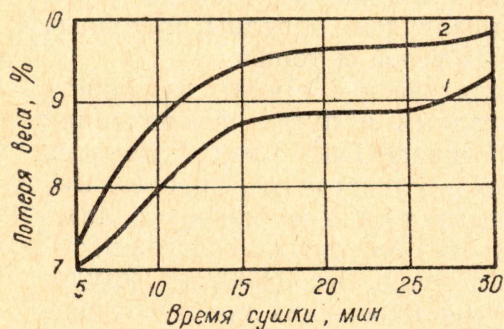
Рис. 3. Зависимость потери веса (в процентах) от времени высушивания образцов торфа: 1 кривая — Бакчарский торф; влажность, определенная стандартным методом — 8,7%; 2 кривая — Таганский торф; влажность, определенная стандартным методом — 9,7%
