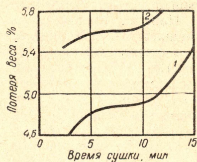
Рис. 2. Зависимость потери веса (в процентах) от времени высушивания образцов бурых углей: 1 — кривая — бурый уголь 1; влажность, определенная стандартным методом — 4,84%; 2 — кривая — бурый уголь 2; влажность, определенная стандартным методом — 5,78%
