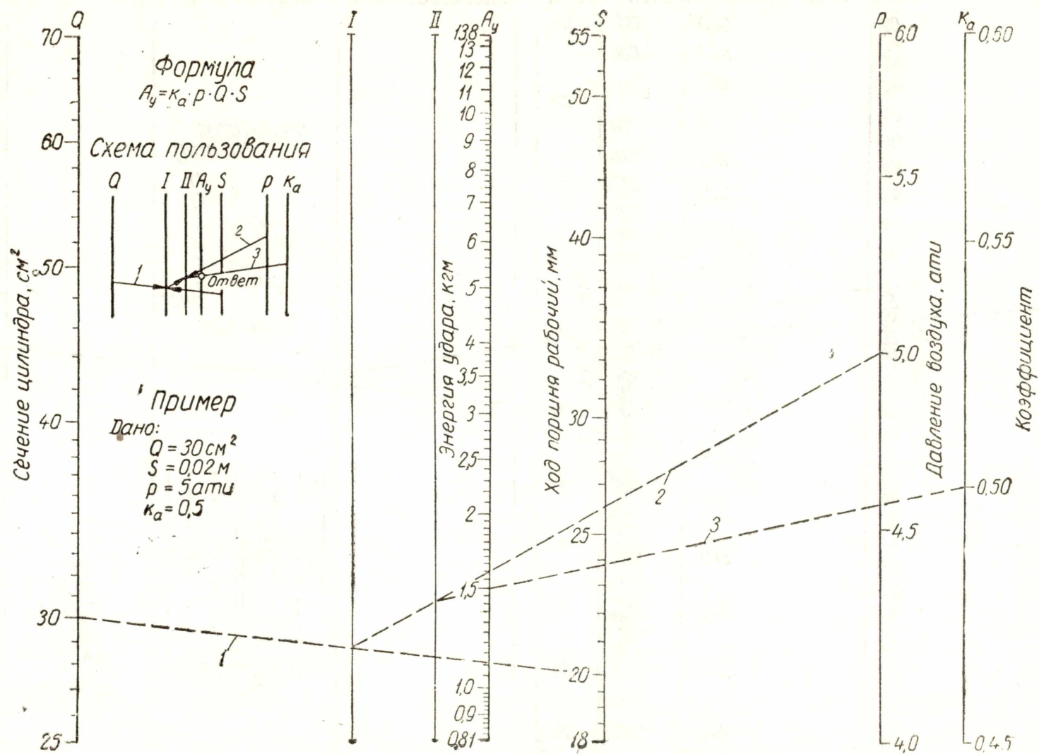
Рис. 1. Номограмма для расчета энергии удара бурильного молотка.
