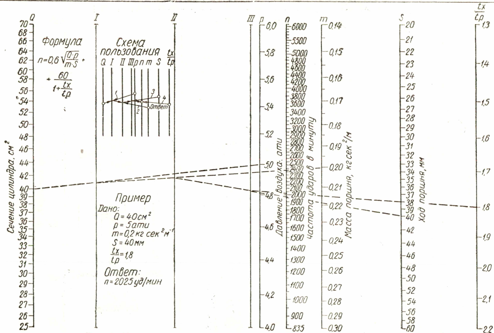
Рис. 2. Номограмма для определения частоты ударов бурильного молотка.
