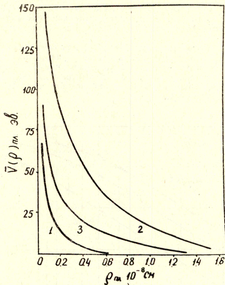
Рис. 3. Средние потенциалы \bar{V}(\rho) пл для плоскостей (100) в KBr
