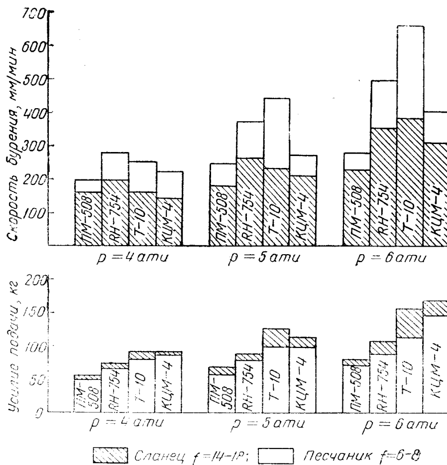
Оптимальные усилия подачи бурильных молотков и соответствующие им скорости бурения коронкой диаметром 46 мм.
