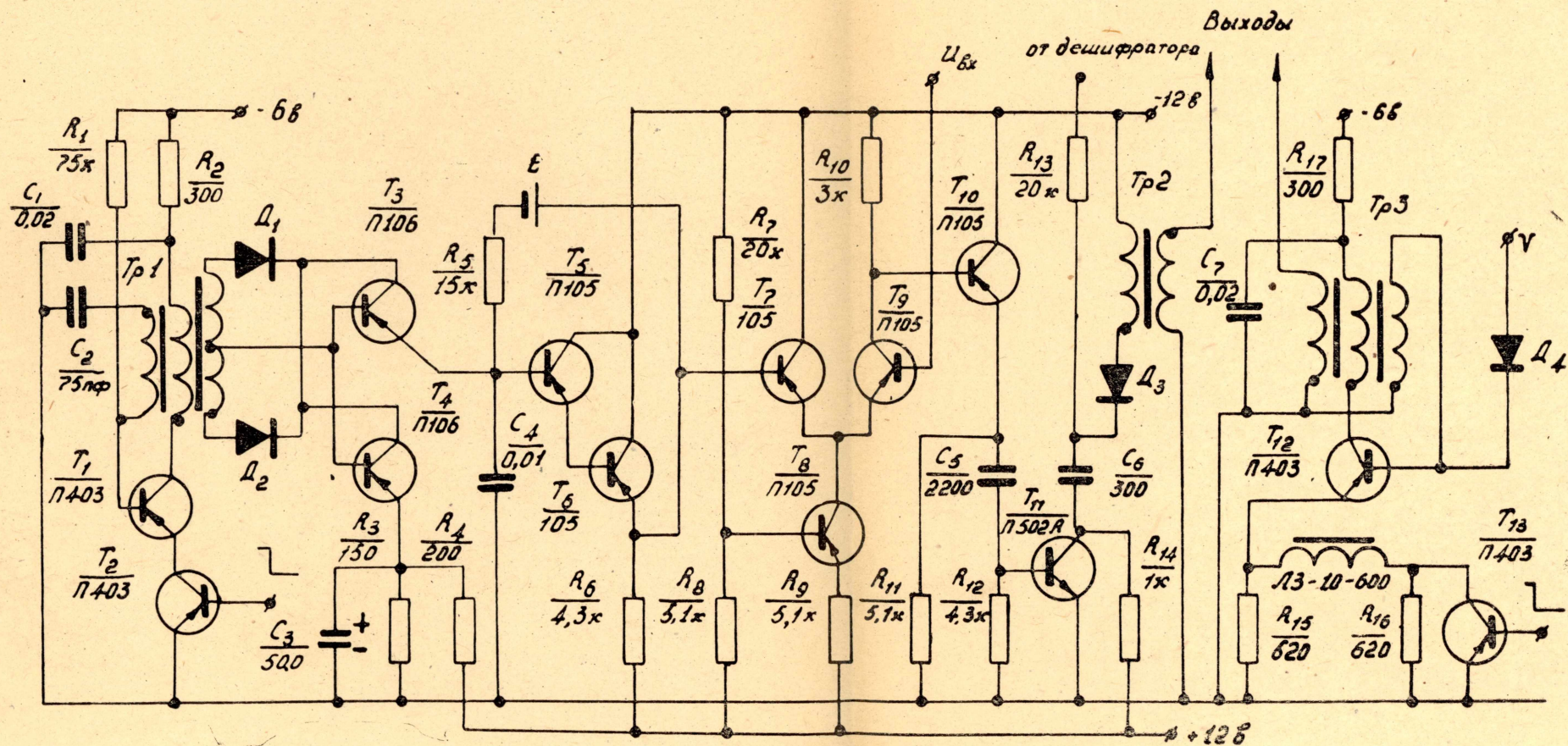
Рис. 1. Принципиальная схема основных узлов преобразователя
