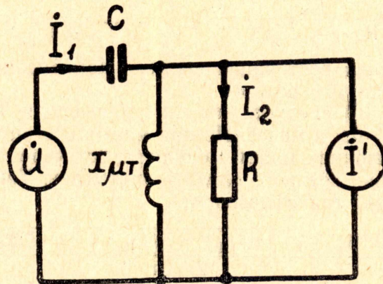
Рис. 2. Схема замещения цепи компаундирования.
