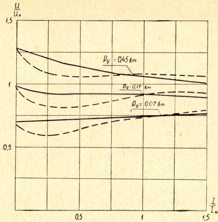
Рис. 3. Внешние характеристики компаундированного БЭМУ-ПЧ. ---- \cos \varphi = 1 , ---- \cos \varphi = 0,8 (инд.).
