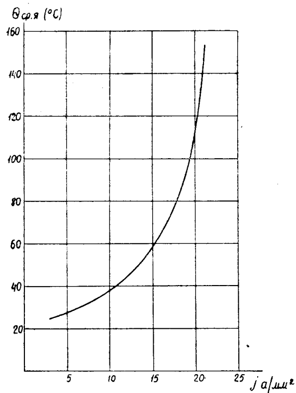
Рис. 1. Зависимость \theta_{\text{ср.я}} = f(j) .
