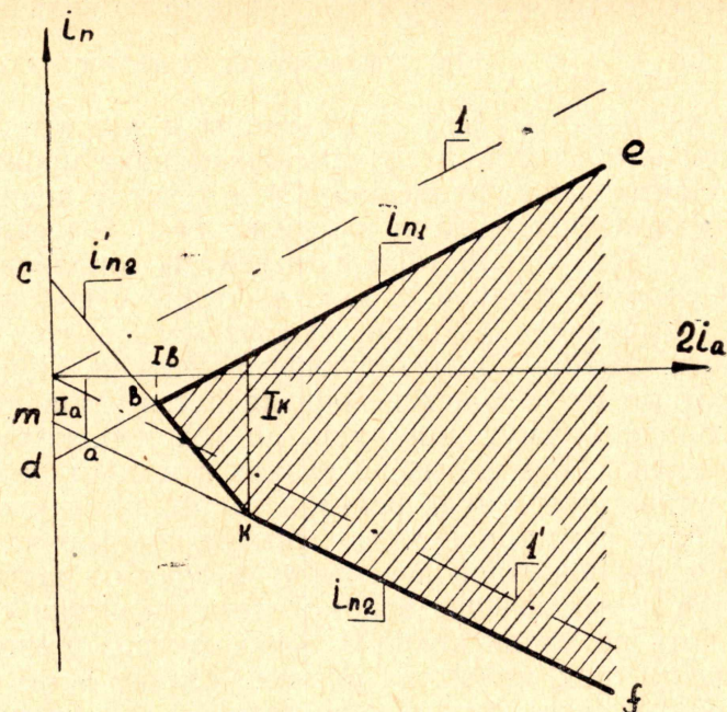
Рис. 2. Теоретическая зона безыскровой работы.
