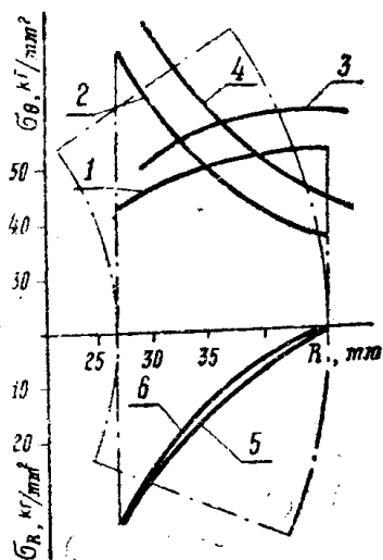
Рис. 1. Эюры напряжений при раздаче стального кольца: 1,3 — эюры окружных напряжений при пластической деформации \delta = 7,5 и \delta = 16\% ; 2,4 — эюры разгрузочных напряжений ( \delta = 7,5 и \delta = 16\% ); 5,6 — эюры радиальных напряжений при пластической деформации и разгрузочных для \delta = 7,5\%
