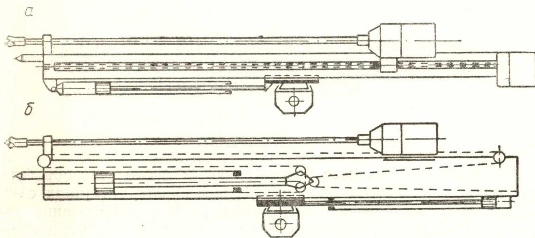
Рис. 2. Принципиальные схемы подающих устройств: а — винтового; б — червячного с цепным удвоителем хода.
