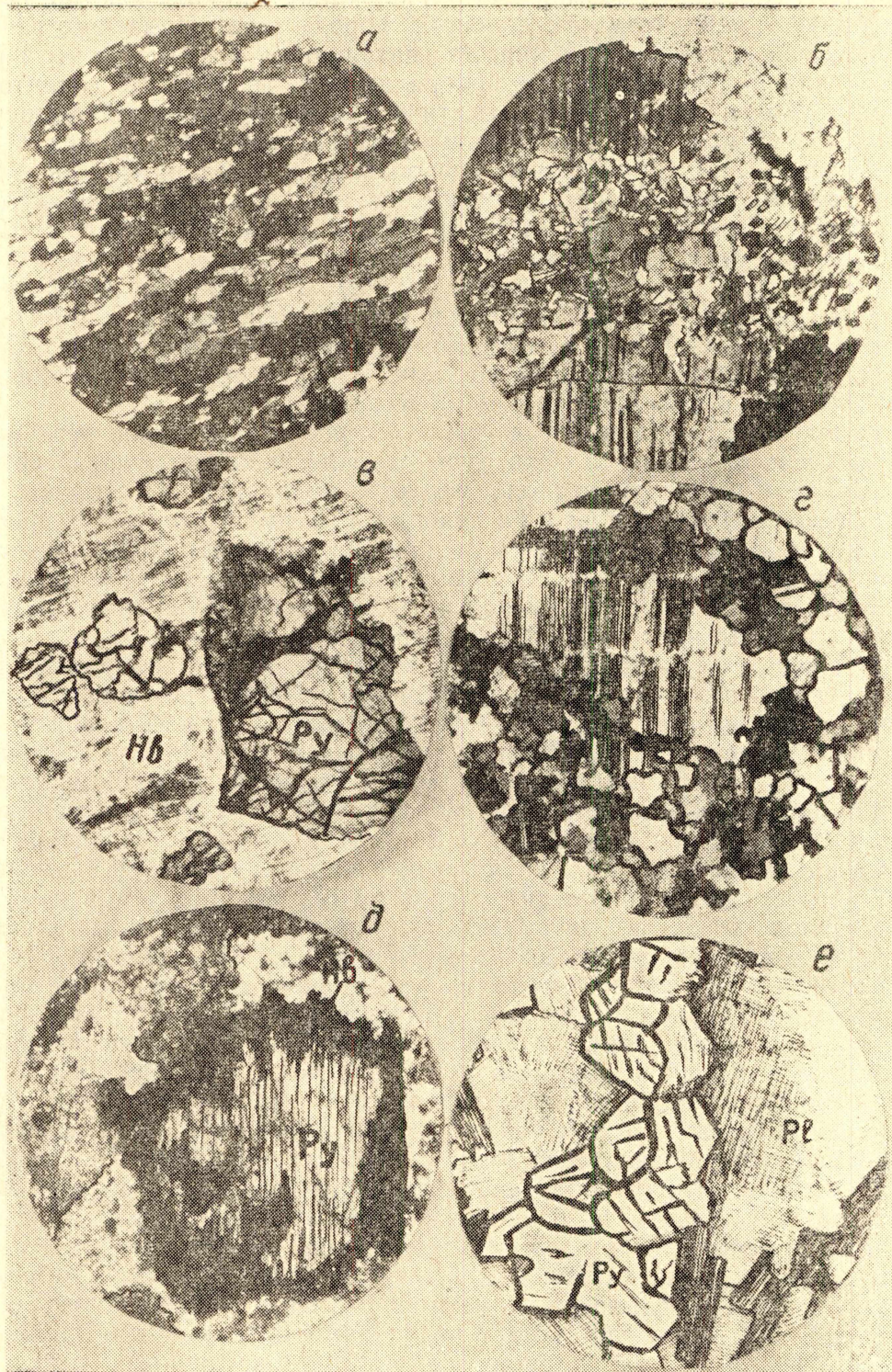
Рис. 2. Микрофотографии петрографических шлифов. а — контактовый амфиболито гнейс; б — бетонная структура в катаклазированном габбро; в — реликты пироксена в зерне уралитовой роговой обманки в амфиболизированном габбро; г — ороговикованное габбро; д — амфиболизация зерна пироксена в амфиболизированном габбро; е — групповое распределение пироксена в гибридных породах Улень-Туимского плутена
