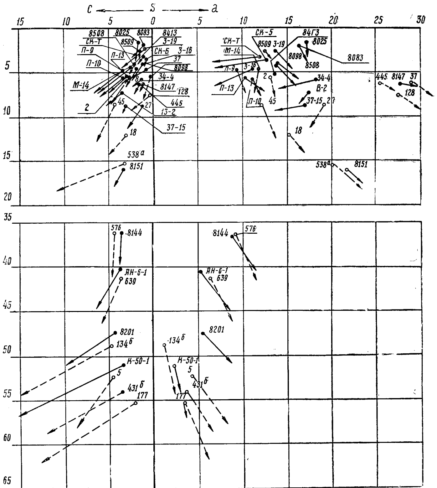
Рис. 2. Диаграмма химических составов магматических пород 8413, 3-19, П-10 — гнейсо-граниты; П-9, П-13 — гранодиориты (р. Уволга); Ск-Б, 3-16 — ногатинские биотитовые граниты Ск-Т, М-14 — ногатинские турмалиновые граниты; 8098 — гранит мелкозернистый (р. Нойба); 8083 — гранит мусковитовый; 8025 — гранит альбитизированный; 8508 — гранит порфировидный; 8509 — гранит мелкозернистый (р. Уволга); 34-4 — сиенит кварцевый; В-2 — сиенит, 37-15 — сиенит-порфир; 8147 — нефелиновый сиенит-порфир; 8151 — цеолитизированный сиенит-порфир; 8144 — бекинкениит; 8201, К-50-1 — жильные кимберлиты; АН-6-1 — оливиновый пироксенит. Средние типы пород по Р. Дэли; 2 — докембрийский гранит Швеции; 45 — гранодиорит, 18 — сиенит; 27 — кератофир; 37 — фойяит; 41 — фонолит; 128 — тингуаит. Некоторые типы горных пород, получившие особое название (по А. Н. Заварицкому): 445 — апачит; 538а — викоит; 576 — бекинкениит; 639 — оливиновый тешенит. Кимберлитовые породы Сибири: 134-Б — жильный кимберлит р. Чапы [6]; 431-Б — жильный кимберлит Чадобецкого поднятия [14]; 177 — жильный кимберлит Якутии [7]; 5 — кимберлитовая брекчия Якутии [7]
