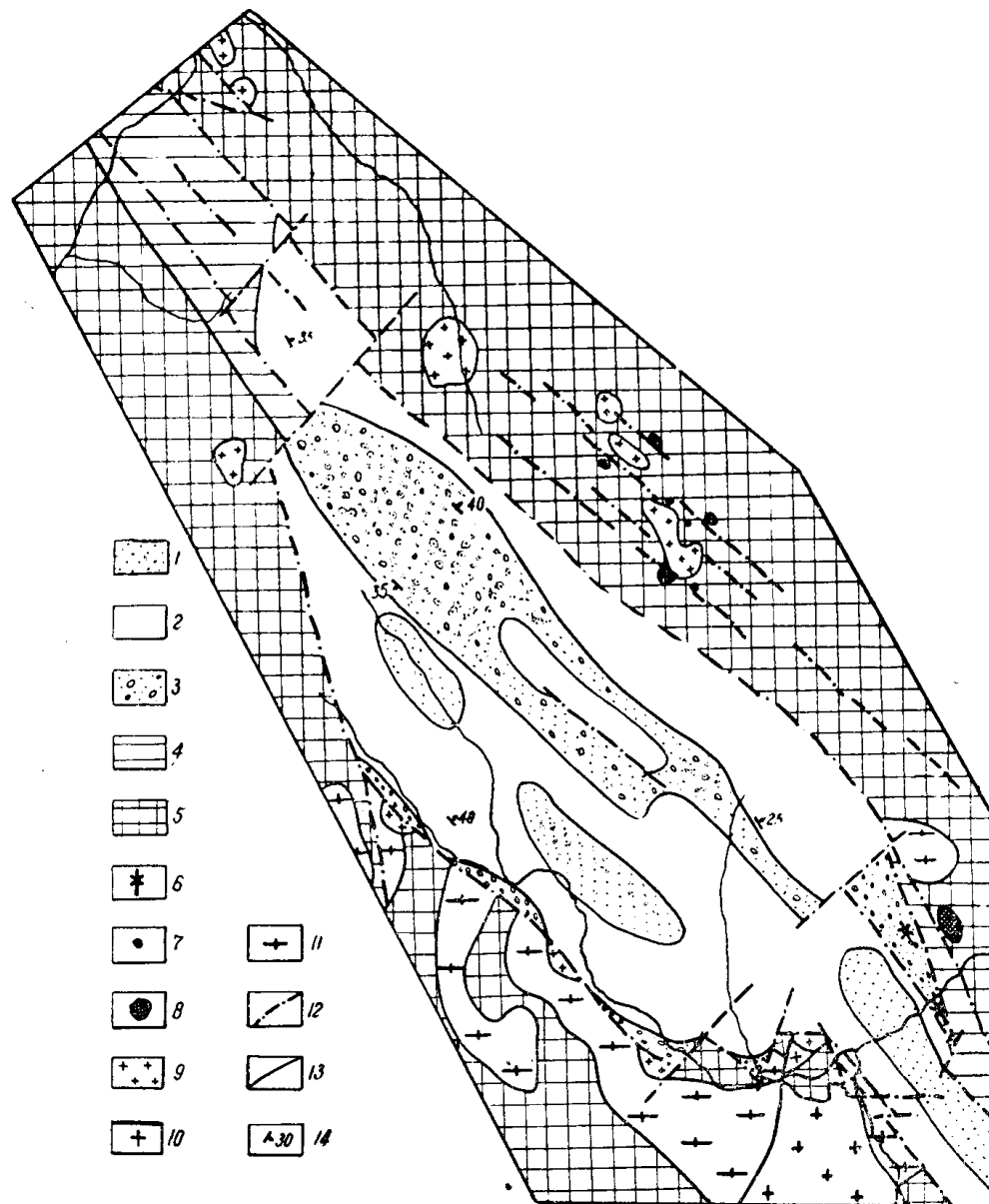
Рис. 1. Схема пространственного размещения интрузивных образований в междуречье Уволги-Чапы. Составил А. Д. Ножкин, 1963 г. Отложения верхнего структурного яруса: 1 — немчанская свита, 2 — чивидинская свита, 3 — лопатинская свита, 4 — образования среднего структурного яруса (удерейская и горбилковская свиты), 5 — метаморфическая толща нижнего структурного яруса (пензенгинская свита), 6 — ультраосновные породы жильного типа, оливниновые пироксениты, 7 — нефелиновые сyenиты (в свалах), 8 — сyenиты, кварцевые сyenиты, сyenит-порфиры, 9 — мелкозернистые граниты, 10 — ногатинские граниты, 11 — гнейсо-граниты; 12 — разрывные нарушения, 13 — геологические границы, 14' — элементы залегания слонстости пород
