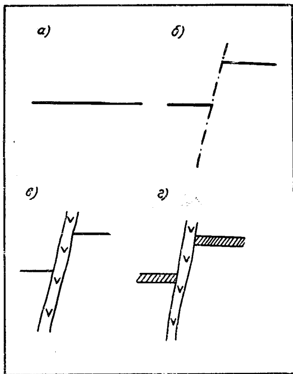
Рис. 1. Этапы формирования ложных пересечений: а — образование неминерализованной рудовмещающей трещины, б — смещение неминерализованной трещины по поперечному дизъюнктиву, в — внедрение дорудной дайки, г — образование рудного тела
