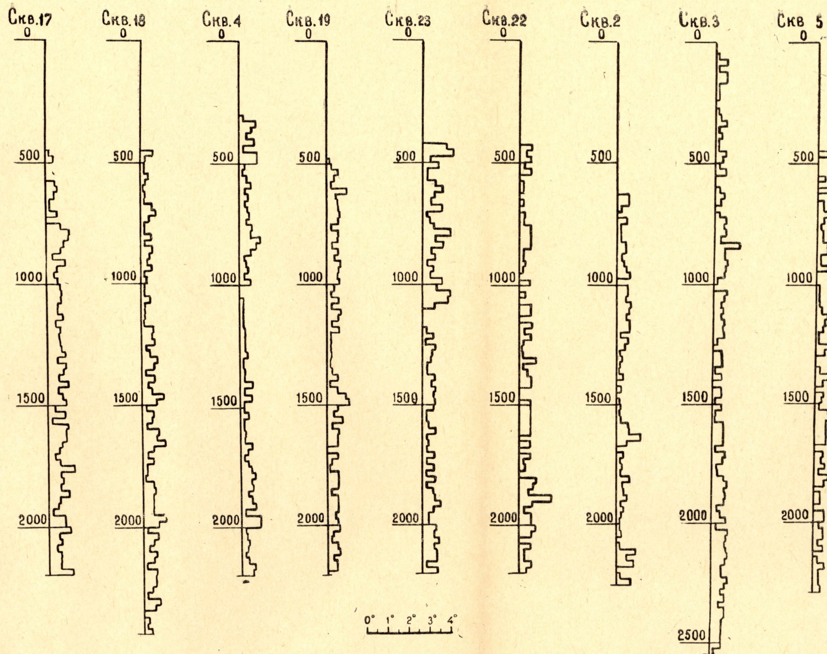
Рис. 2. Интенсивность искривления скважин Александровской нефтеразведки. Вертикальные прямые символизируют оси скважин, цифры слева от них показывают глубину в метрах. Величины интенсивности даны в градусах на 25 метров, масштаб общий в нижней части рисунка
