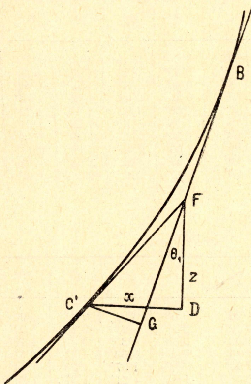
Рис. 1. Взаимоотношение между касательными, проведенными к оси скважины в двух смежных точках замера
