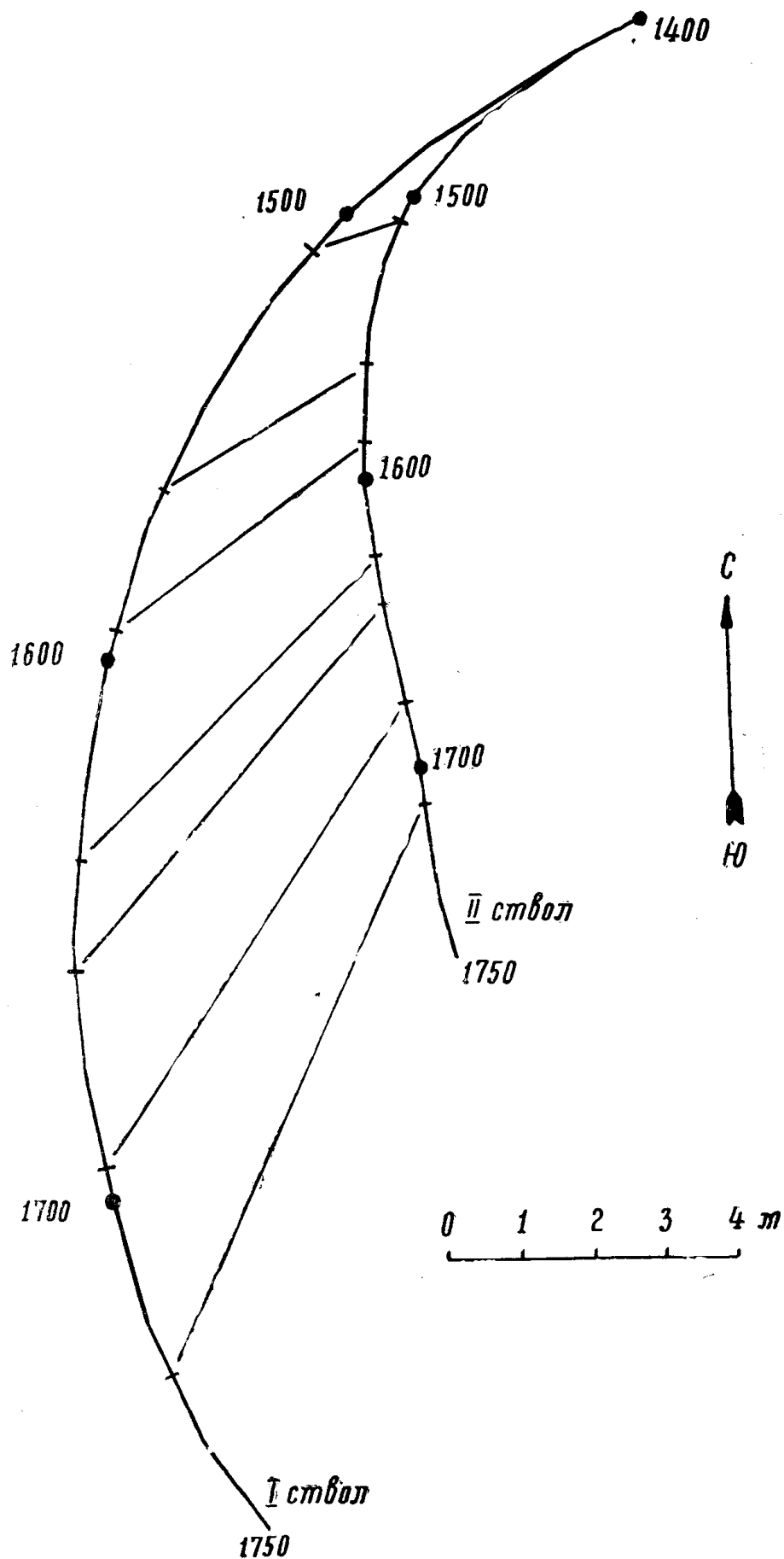
Рис. 1. Горизонтальная проекция разветвленной части двухзабойной скважины. Цифрами обозначены номинальные глубины (глубины при замере по стволу) в точках, отмеченных кружками. Короткие поперечные линии показывают места точек встреч ответвлений скважины с кровлями проходимых пластов. Прямые линии между ними — прямые косых сечений
