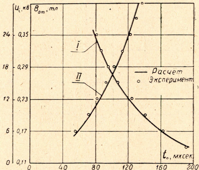
Рис. 3. Оптимальная фаза инжекции: 1 — при изменении индукции на равновесной орбите, U_i = 44 кВ; 2 — при изменении напряжения инжекции, B_{om} = 0,23 мВ.
