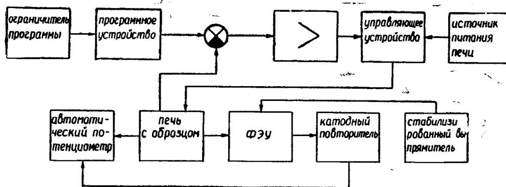
Рис. 1. Блок-схема установки термолюминесценции
