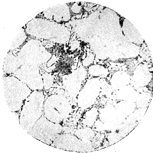
Рис. 5. Микроструктура литой стали P18 с 1,3% C; \times 600 (травитель: 10 г K_3(CN)_6 , 10 г KOH на 100 мл воды)
