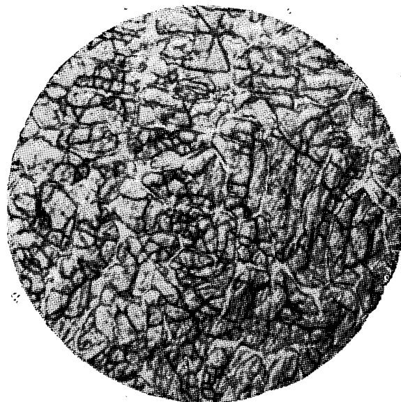
Рис. 1. Микроструктура стали плавки 15 в литом состоянии. × 450
