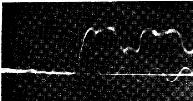
Рис. 1. Оциллограмма импульса с пробоем на плоской части. Частота градуировочных колебаний 100 мгги
