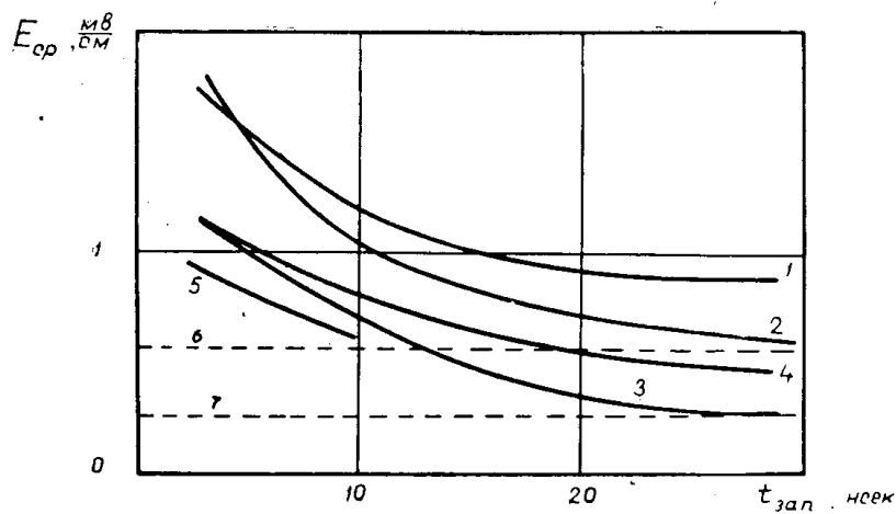
Рис. 2 а, б. Зависимость средней пробивной напряженности от времени приложения напряжения для полистирола 1, полиэтилена 2, органического стекла 3, фторопласта-4 (4) и поливинилиденхлорида 5, 6 и 7 — средние пробивные напряженности для полистирола и органического стекла при экспозиции напряжения 6 \cdot 10^{-6} сек.
