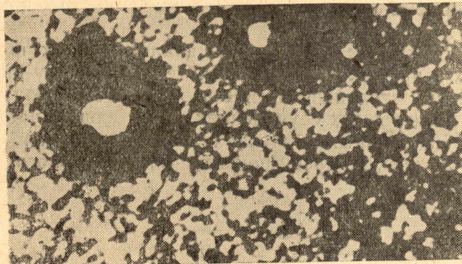
Рис. 3. Пленка SiO 2 , напыленная без сепаратора на скол NaCl. Увеличение \times 24000 . Видно две поры
