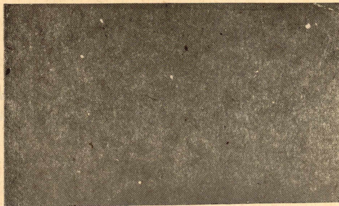
Рис. 2. Пленка SiO 2 , напыленная с сепаратором на стекло. Увеличение \times 400 , темнопольное изображение
