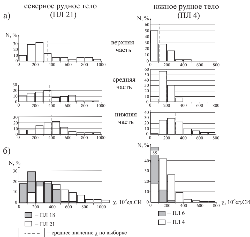
Рис. 5. Изменение магнитной восприимчивости руд арсенопирит-пирротиновой ассоциации по: а) восстанию и б) простиранию
