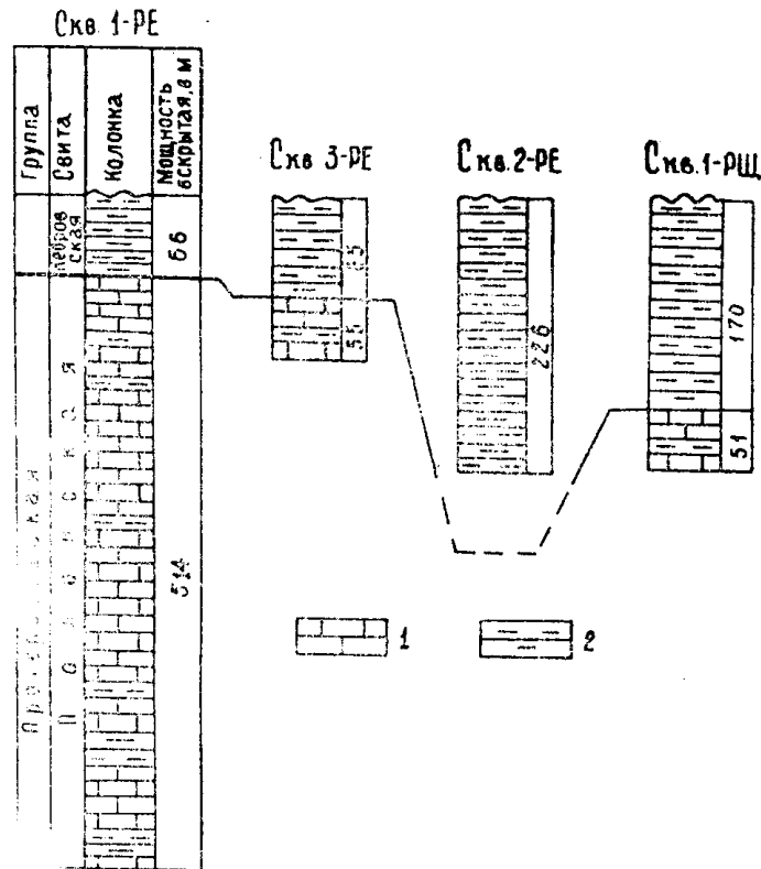
Рис. 2. Схема сопоставления докембийских образований в районе поселка Ермаково: 1 — мраморизованные известняки, 2 — сланы
