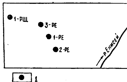
Рис. 1. Обзорная схема района работ: 1 — глубокие разведочные скважины
