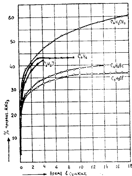
Рис. 1. Скорость нитрования бензола, толуола, иодбензола, бромбензола и хлорбензола.
