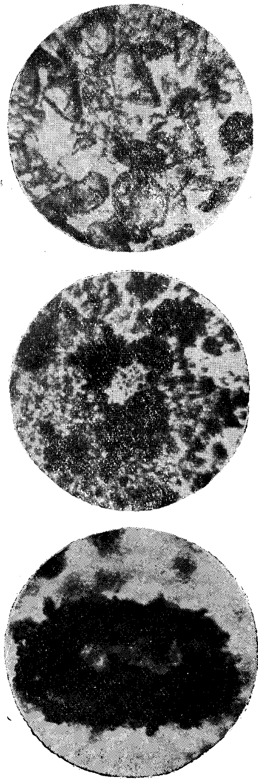
Рис. 1. Микрофотография смеси циркона с карбонатом кальция, 400х: а — необожженной, б — обожженной при 1100°С, в — обожженной при 1300°С
