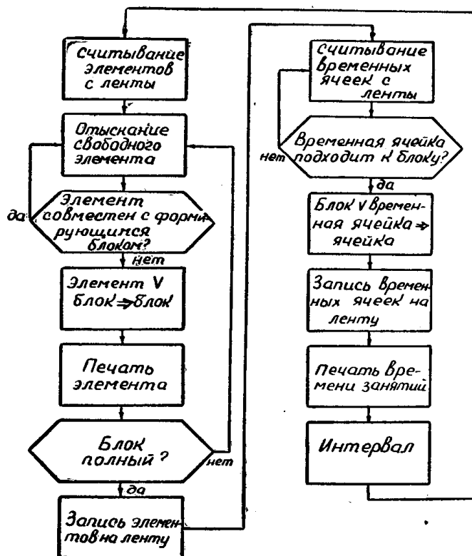
1. Краткая блок-схема программы
