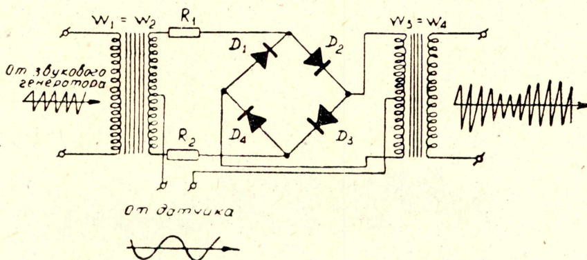
Рис. 3. Схема модулятора
