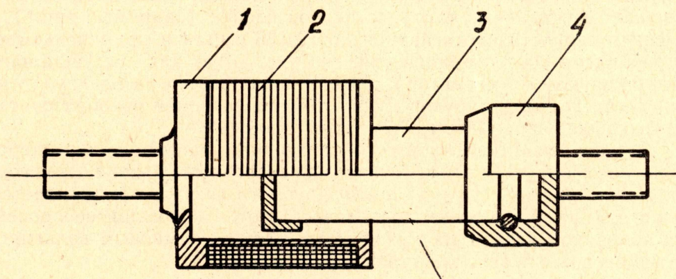
Рис. 2. Магнитоэлектрический датчик: 1 — корпус, 2 — обмотка, 3 — магнит, 4 — оправка
