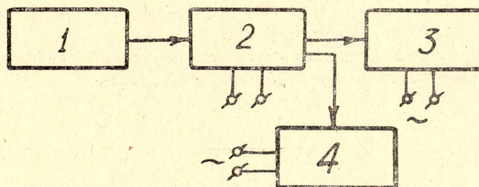
Рис. 4. Структурная схема для анализа колебаний пневматических молотков
