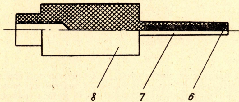
Рис. 1. Индуктивный датчик: 1 — контактный лепесток, 2 — заклепка, 3 — измерительная обмотка, 4 — генераторная обмотка, 5 — каркас, 6 — пробка, 7 — ферритовый стержень, 8 — оправка
