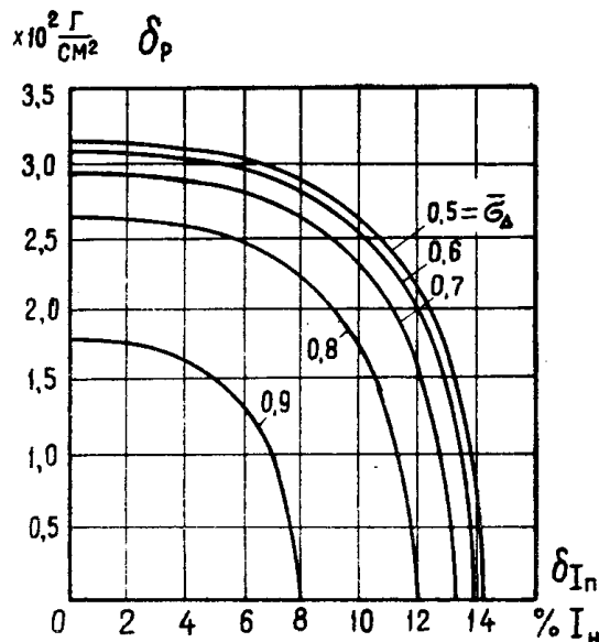
Рис. 1. Система допусков для машин третьего габарита серии П при допустимом искрении 1 балла и вероятности брака 0,0027
