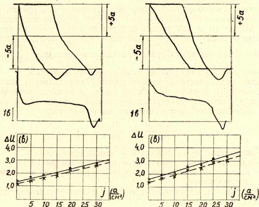
Рис. 1. Динамические вольтамперные характеристики скользящего контакта при коммутации различных секций одного паза катодно-поляризованной щеткой: опытные — сплошные линии, расчетные — штриховые линии
