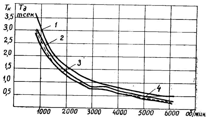
Рис. 3. Зависимости T_{\kappa} и T_{\partial} от скорости вращения.
