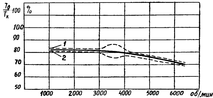
Рис. 5. Зависимость \frac{T_d}{T_k} 100=f(n) для щетки ЭГ-14. 1—2 область рассеивания
