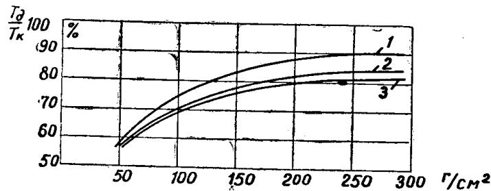
Рис. 7. Зависимость \frac{T_{\partial}}{T_k} \cdot 100 от нажатия при n = 2500 об/мин. 1 — ЭГ-4Э; 2 — ЭГ-14; 3 — ЭГ-74
