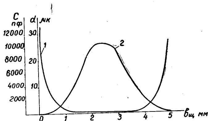
Рис. 9. Кривые распределения зазора и емкости между щеткой и ламелью. 1 — распределение зазора под щеткой; 2 — распределение емкости контакта
