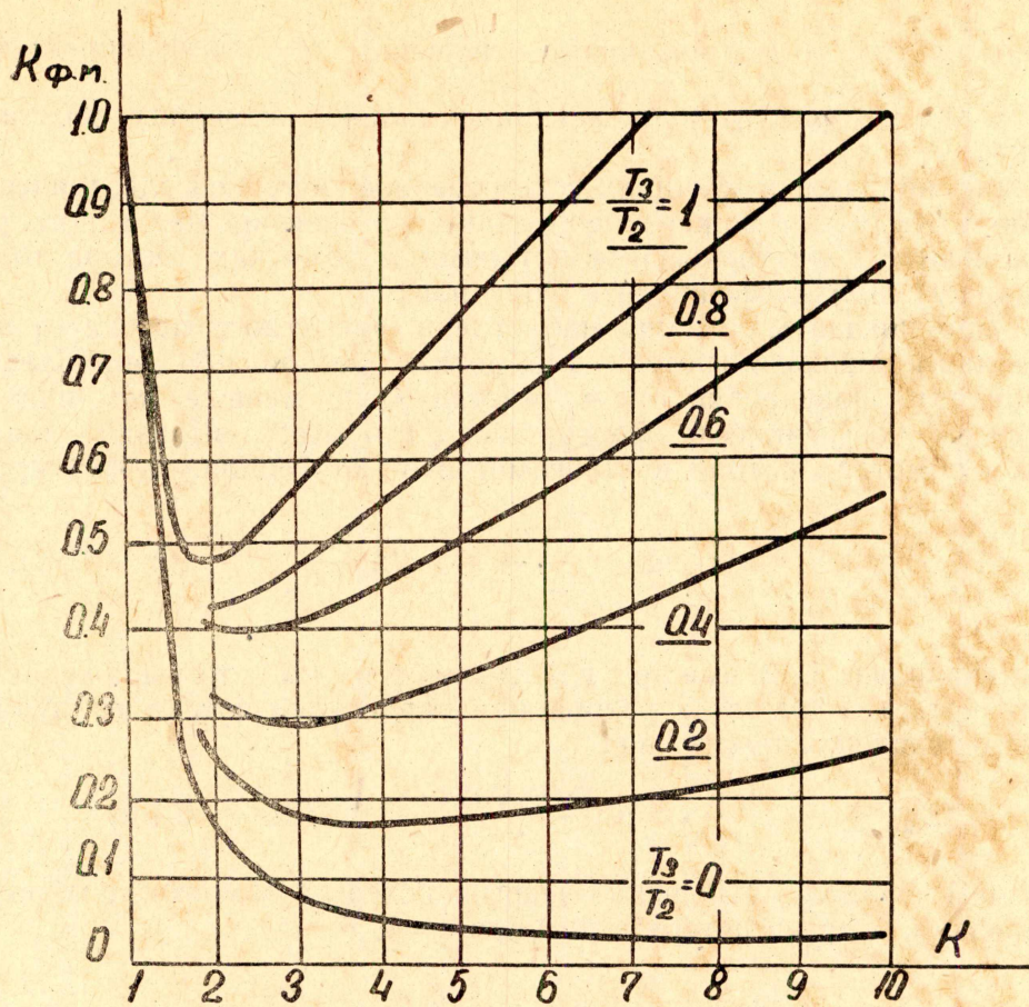
Рис. 4. Зависимость K_{fm} от коэффициента форсировки
