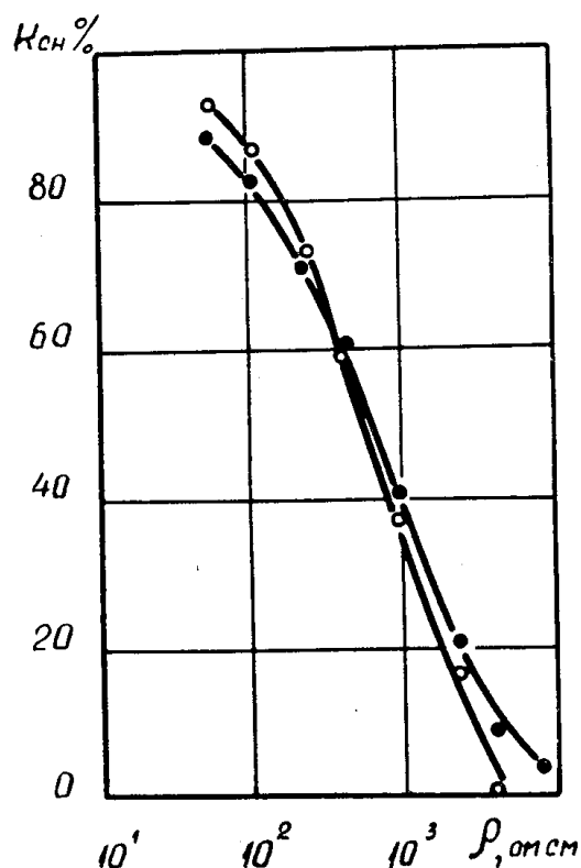
Рис. 2. Зависимость коэффициента снижения амплитуды напряжения от удельного сопротивления воды:
