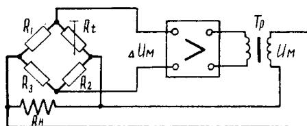
Рис. 1. Схема стабилизатора температуры
