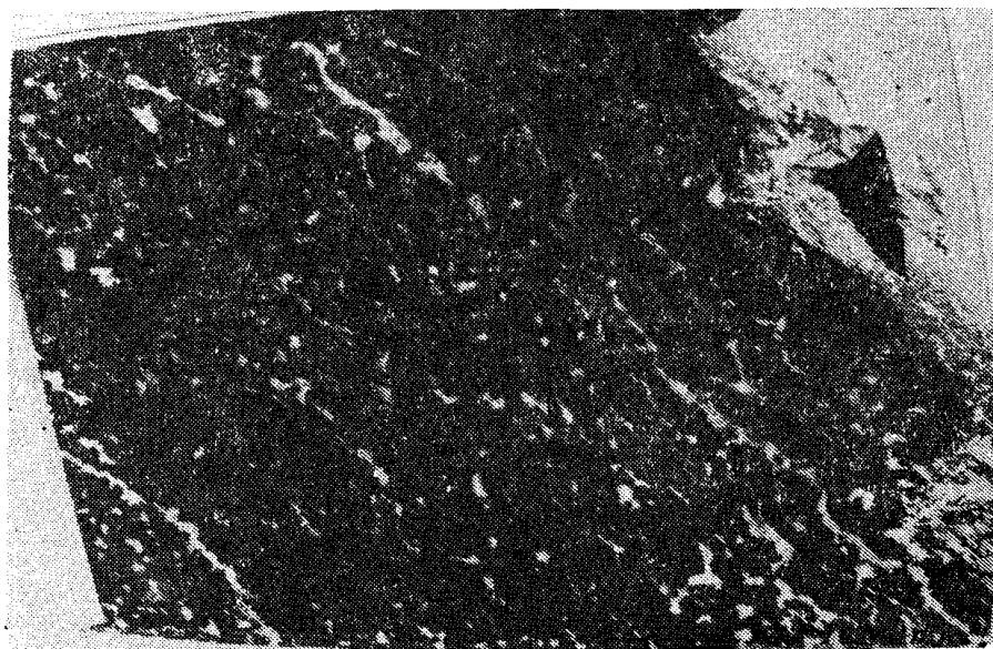
Рис. 2. Палеомикроцистисовый доломит.
