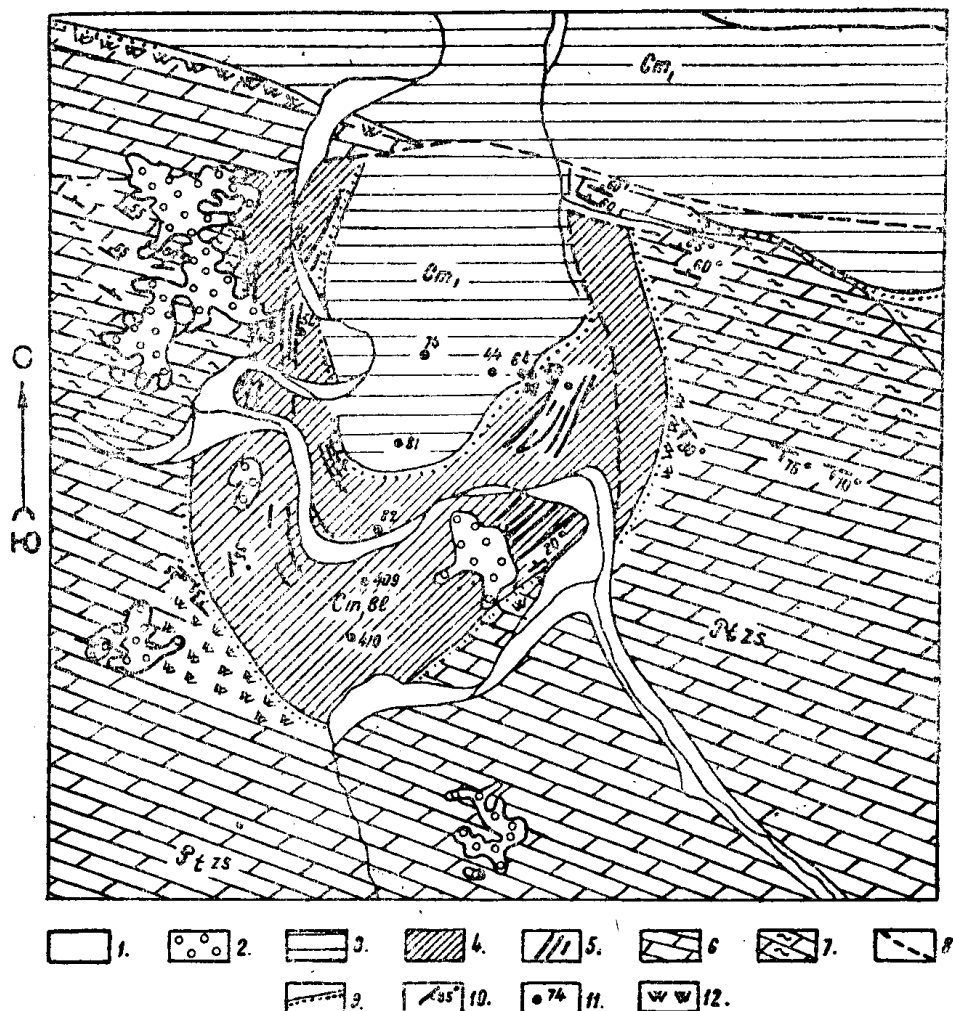
Рис. 1. Схематическая геологическая карта участка Белка в Горной Шории: 1 — четвертичные отложения; 2 — фосфориты континентальные мезо-кайнозойского возраста; 3 — карбонатные отложения нижнего кембрия. Белкинская свита низов нижнего кембрия; 4 — различной степени фосфатности известняки, 5 — фосфориты пластовые. Западносибирская свита позднего докембрия; 6 — доломиты массивные водорослевые, реже брекчиевые и оолитовые; 7 — доломиты с палеомикроцистисами; 8 — дизъюнктивные нарушения; 9 — стратиграфические границы между подразделениями докембрия и кембрия; 10 — элементы залегания слоистости; 11 — скважины; 12 — микрокварциты метасоматического происхождения.
