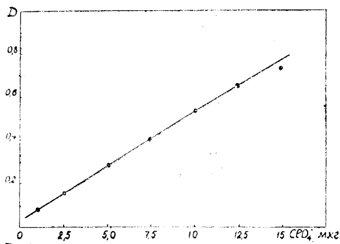
Рис. 2. Калибровочный график. Объем колбы 25 мл, кювета с толщиной слоя 2 см, светофильтр № 8, концентрация реактива 0,4%.
