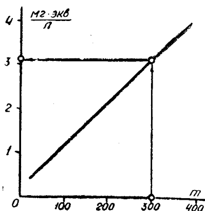
Рис. 1. Градуировочная кривая для определения временной жесткости томской воды по показаниям интерферометра (кювета 80 мм).
