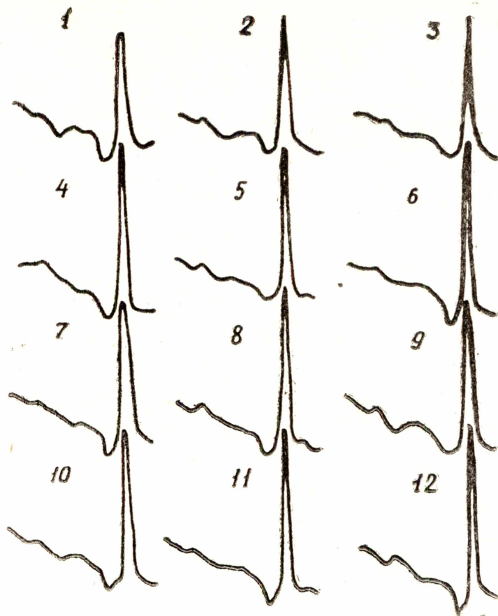
Рис. 1. Дифференциально-термические кривые. Количество добавки \text{TiO}_2 , %: 1 — без добавки, 2 — 0,02; 3 — 0,04; 4 — 0,06; 5 — 0,08; 6 — 0,1; 7 — 0,125; 8 — 0,25; 9 — 1; 10 — 2; 11 — 3; 12 — 4.
