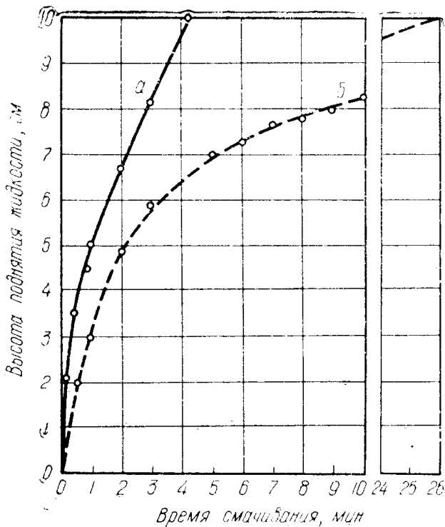
Рис. 1. Зависимость высоты подъема воды от времени: б — исходного, содержащего пленку гуминовых веществ; а — песка, обработанного 1% раствором NaOH.
