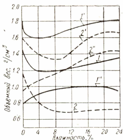
Рис. 1. Зависимость между влажностью материалов и изменением их объемного веса: 1 — кварцевый песок без уплотнения, 2 — маршалит без уплотнения, 1' — кварцевый песок при вибрационном уплотнении, 2' — маршалит при вибрационном уплотнении, 1'' — степень уплотнения кварцевого песка, 2'' — степень уплотнения маршалита (ординаты этих кривых есть разность ординат кривых 1', 2' и 1, 2).
