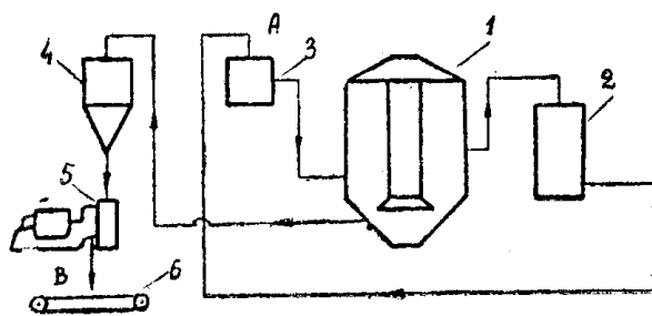
Рис. 1. Технологическая схема сатураторного цикла: 1 — сатуратор, 2 — циркуляционная кастрюля, 3 — кастрюля обратных токов, 4 — кристаллоприемник, 5 — центрифуга, 6 — транспортер. А — место подачи добавки, В — место отбора проб
