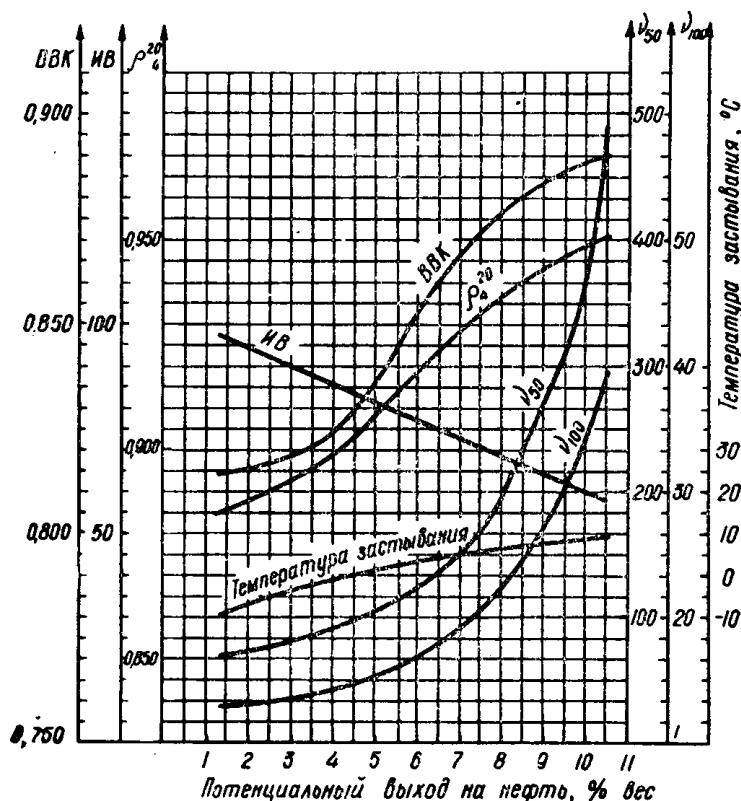
Рис. 2. Кривые зависимости качества масел от глубины адсорбционного разделения остатка выше 450°C
