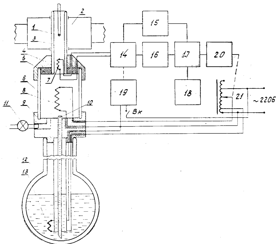
Рис. 1. Схема установки
