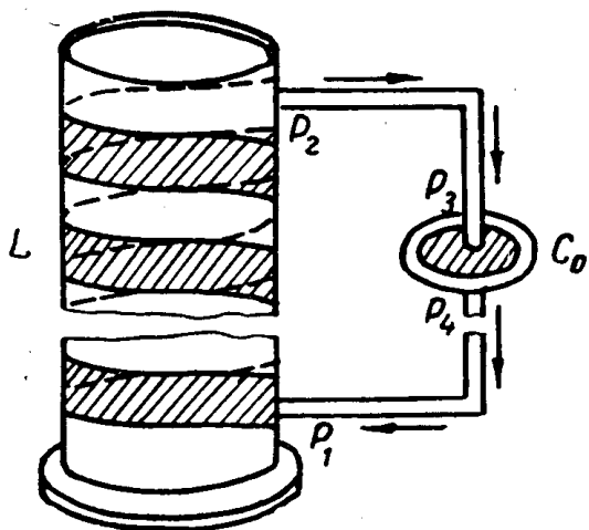
Рис. 1. Катушка индуктивности с емкостью
