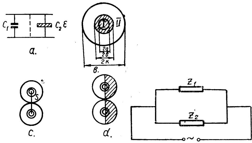
Рис. 5. Схемы нескольких вариантов расчета собственной емкости катушки
