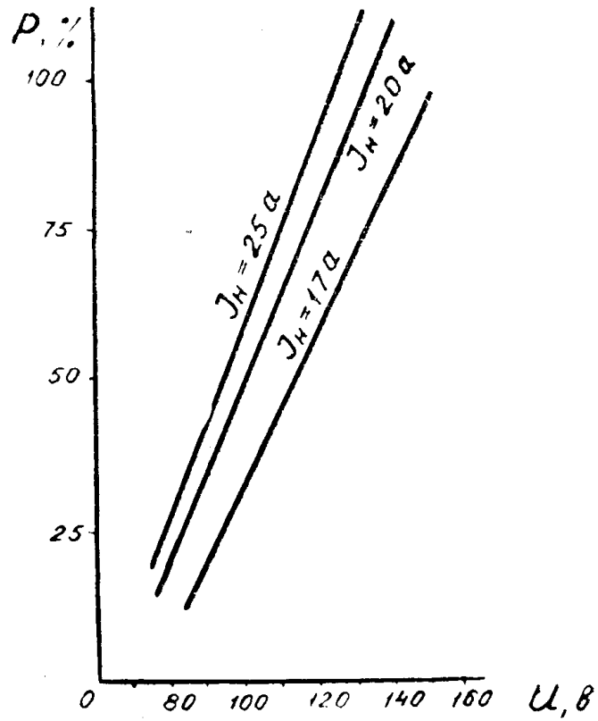
Рис. 3. Вольтамперные характеристики
