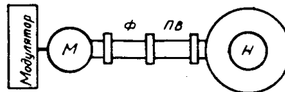
Рис. 1. Блок-схема генератора
