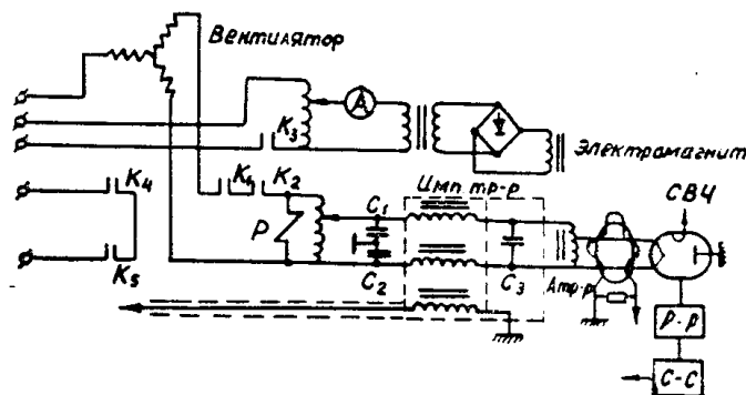
Рис. 2. Электрическая схема цепей генератора
