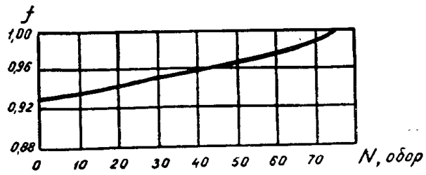
Рис. 4. Диапазон изменения частоты генератора при перестройке
