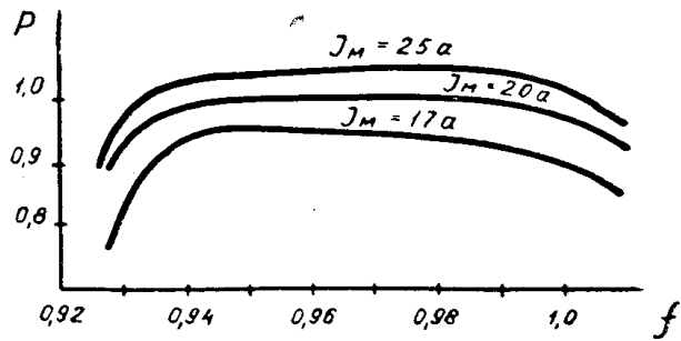
Рис. 5. Зависимость генерируемой мощности от частоты
