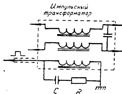
Рис. 8. Включение корректирующей цепи
