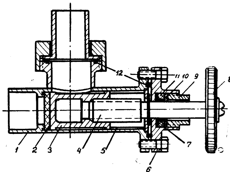
Рис. 2. Вентиль: 1 — корпус вентилья, 2 — фторопластовый диск, 3 — клапан, 4 — винт, 5 — стопорная втулка, 6 — фланец, 7 — фторопластовая втулка, 8 — маховичок, 9 — гайка, 10 — шайба, 11 — резиновая прокладка
