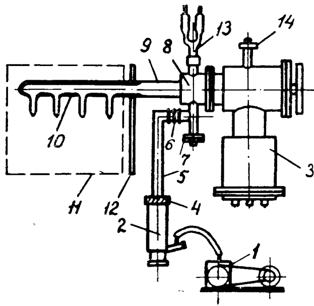
Рис. 1. Схема вакуумной системы откачного поста: 1 — механический насос РВН-20, 2 — диффузионный насос ЦВЛ-100, 3 — титановый насос, 4 — ловушка, 5 — трубопровод, 6 — сильфон, 7 — вентиль предварительной откачки, 8 — колпак, 9 — коваровая трубка, 10 — стеклянная гребенка, 11 — печь, 12 — экран, 13 — манометрические лампы ЛТ-2 и ЛМ-2, 14 — датчик ММ-13
