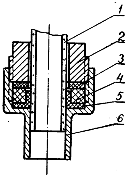
Рис. 4. Резино-фторопластовое уплотнение манометрических ламп: 1 — лампа, 2 — гайка, 3 — шайба, 4 — резиновая прокладка, 5 — фторопластовая втулка, 6 — корпус
