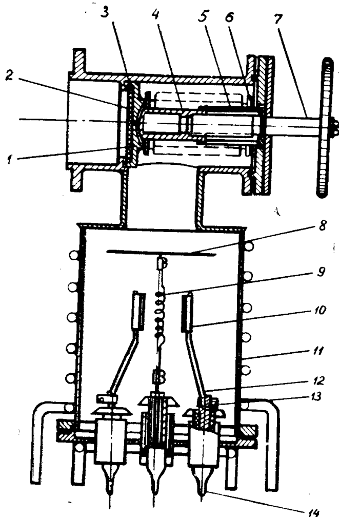
Рис. 3. Схема титанового насоса: 1 — шайба, 2 — фторопластовый диск, 3 — клапан, 4 — нажимная втулка, 5 — стопорная втулка, 6 — сильфон, 7 — винт, 8 — экран, 9 — катод, 10 — анод (коллектор), 11 — корпус насоса, 12 — молибденовый держатель, 13 — стяжная лента, 14 — металлокерамический ввод
