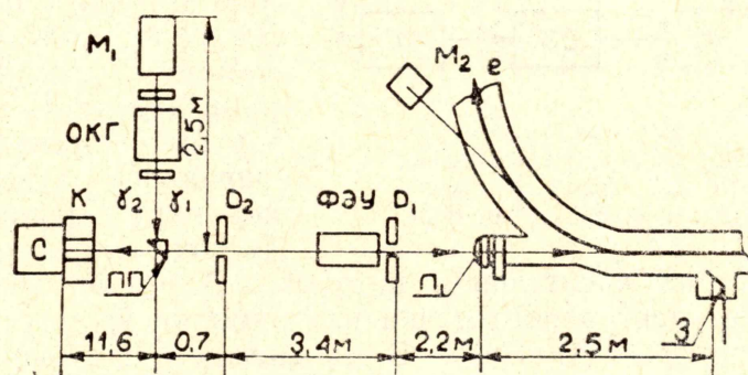
Рис. 1. Схема расположения экспериментального оборудования. L_1 — фокусирующая линза, ВКУ — вакуумная камера ускорителя, M_1 — монитор электронного пучка, D_1 и D_2 — подвижные диафрагмы, ПП — поворотная призма, ОКГ — рубиновый лазер, M_2 — монитор излучения лазера, К — коллиматор, С — спектрометр
