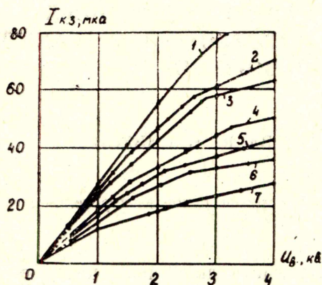
Рис. 1. Характеристики к. з., полученные при следующих величинах зазора ротор-статор: 1. 0,2 мм; 2. 0,4 мм; 3. 0,6 мм; 4. 0,8 мм; 5. 1,5 мм; 6. 3,0 мм; 7. 4,0 мм
