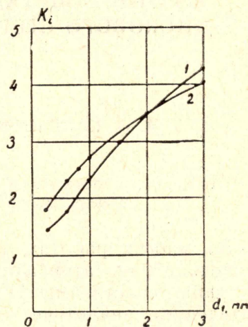
Рис. 3. Зависимость коэффициента естественной перезарядки от величины воздушного зазора: 1 — экспериментальная; 2 — расчетная
