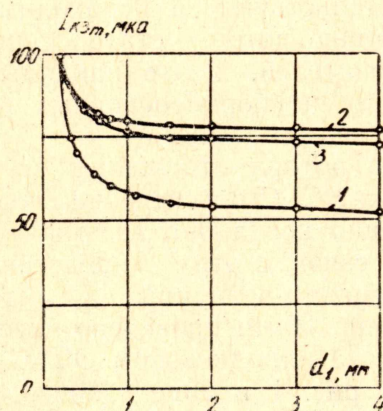
Рис. 1. Зависимости максимального тока к. з. от величины зазоров ротор-статор однодискового ЭСГС
