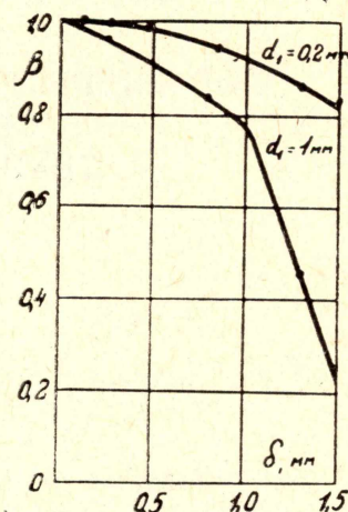
Рис. 3. Зависимости максимального тока к. з. от величины зазора ротор-щеточка при различных зазорах ротор-статор
