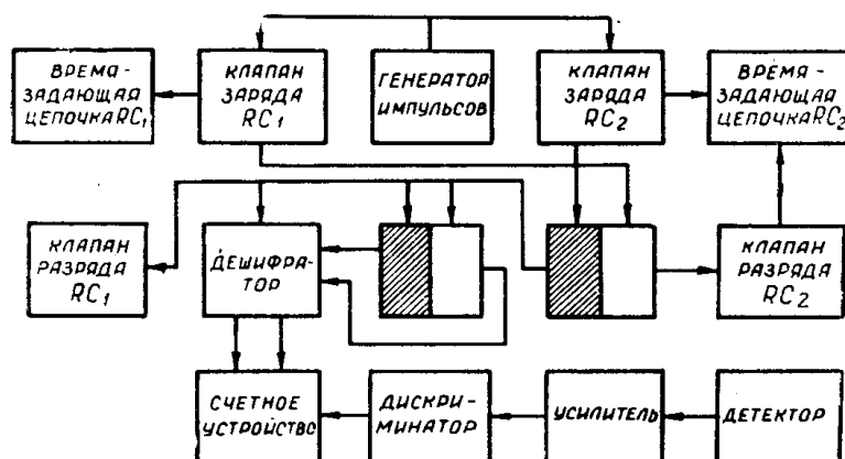
Рис. 1. Блок-схема прибора
