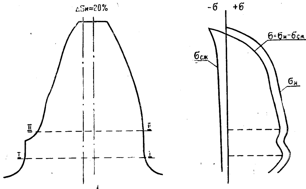
Рис. 1. Профиль зуба, изношенного на 20%, и эпюры напряжений
