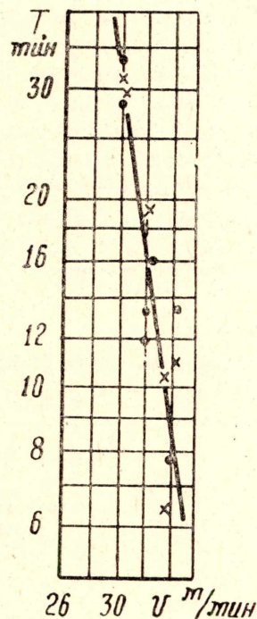
Рис. 2. Стойкость T в зависимости от скорости резания V резцов из стали Р12 с различными режимами отпуска: ● — обычного, х — кратковременного
