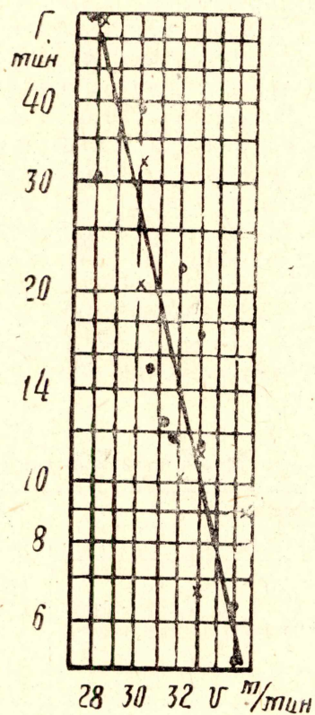
Рис. 1. Стойкость T в зависимости от скорости резания V резцов из стали Р18 с различными режимами отпуска: ● — обычного, х — кратковременного
